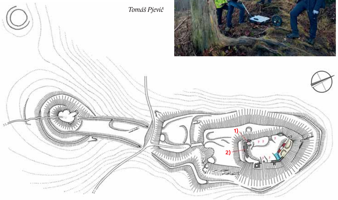
Půdorys hradu
